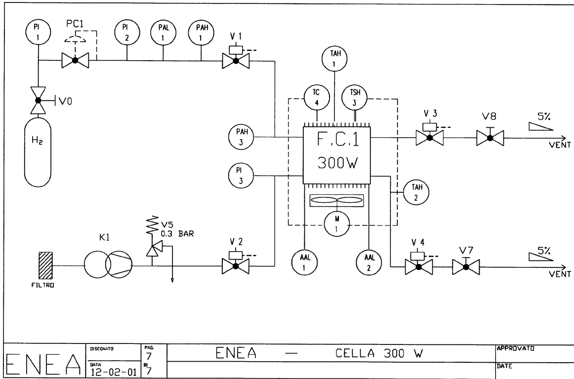
Fig. 2. PI&D.
